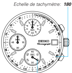
Aiguille des secondes du CHRONO: 20 secondes
